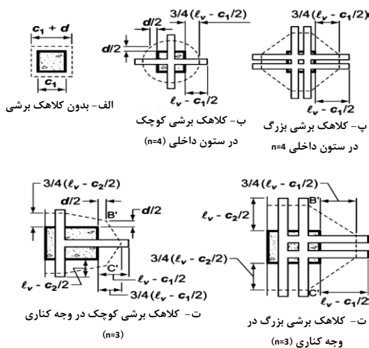
شکل ۸-۸ موقعیت مقطع بحرانی در کلاهک برشی
