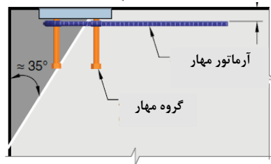
(ب) آرماتور مهار سنجاقی برای مهار برش
