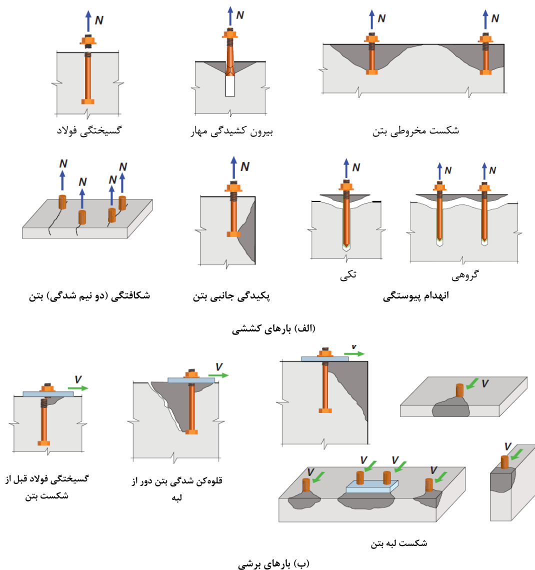
شکل ۳-۱۸ انواع حالات شکست مهارها در کشش و برش
