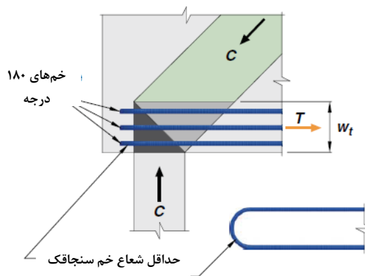
شکل ۱۲-۲۲ یک گره C-T-C که با سنجاک‌های خم شده ۱۸۰ درجه مهار شده‌اند
