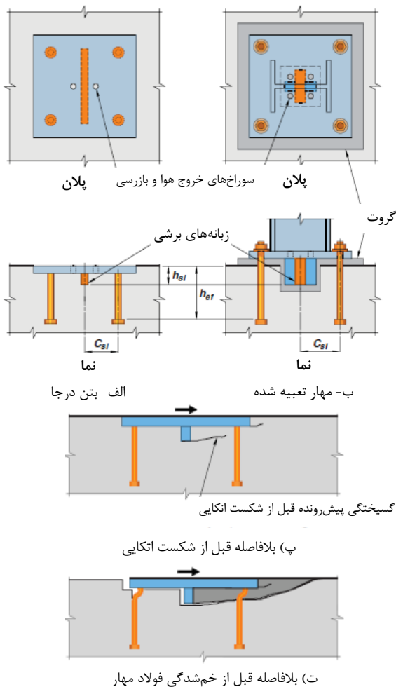
شکل ۱۱-۱۸ شکست اتکایی و خمش شدگی مهار برای صفحه جاگذاری شده زبانه برشی
