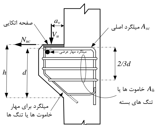
(ب) آرماتورگذاری نشیمن
