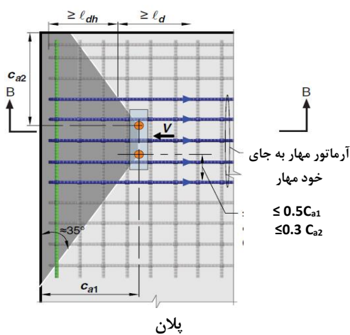
(پ) آرماتور مهار و آرماتور گوشه برای برش
