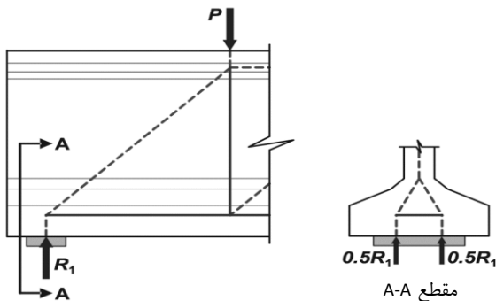
شکل ۲۲-۱۶ تبدیل مدل خرپای دوبعدی در جان تیر I شکل به مدل سه‌بعدی در بال تیر
