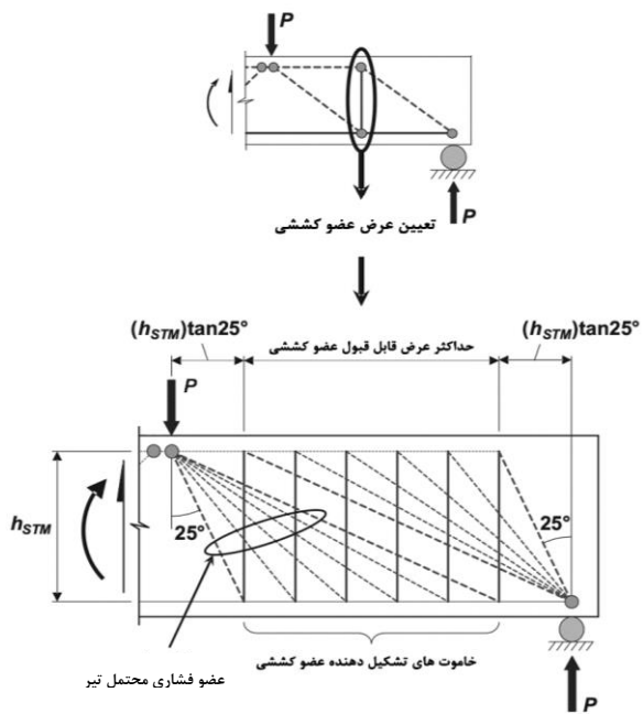
شکل ۲۲-۱۷ نحوه تعیین عرض اعضای کششی قائم داخلی در مدل خرپایی تیر عمیق
