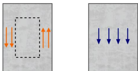
تنش‌های برشی ناشی از برش ب - مقطع توپر
