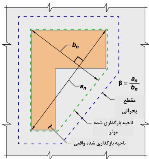
شکل ۸-۵ مقدار \beta برای سطح زیر بار غیر مستطیلی
