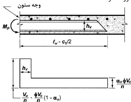
شکل ۷-۸ برش ایده‌آل در کلاهدک برشی
