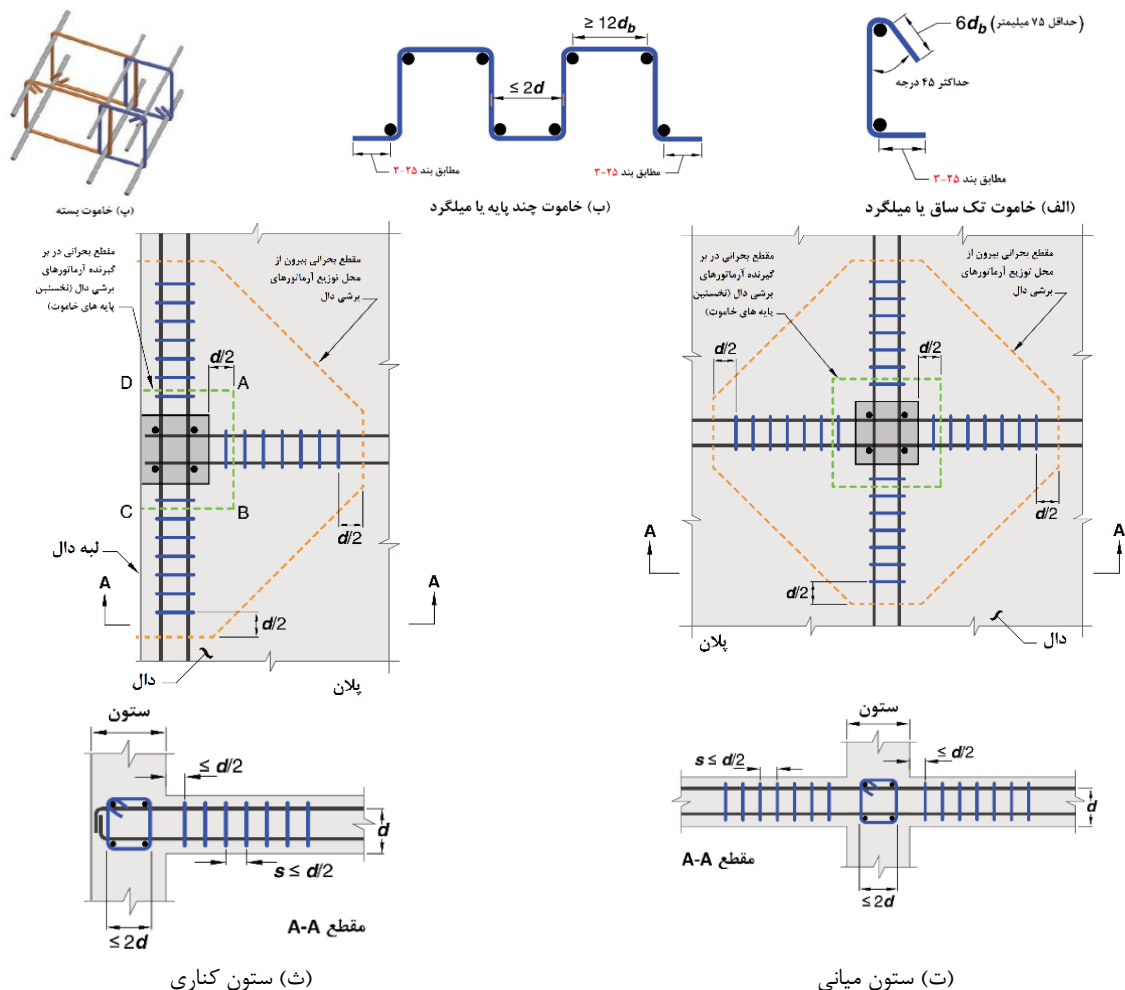
شکل ۷-۱۰ نحوه تنظیم و توزیع آرماتورهای برشی دال (خاموت‌ها)
