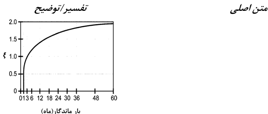
شکل ۱-۱۹ ضرایب افزایشده تغییر مکان های بلند مدت
