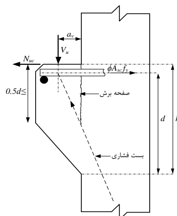
(الف) انواع تلاش‌ها در یک نشیمن
