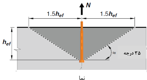
نما الف- شکست مخروطی بتن در کشش
