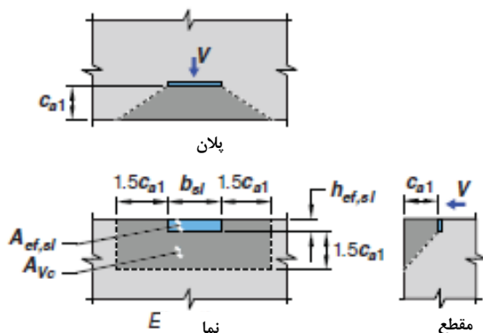
شکل ۱۸-۱۳ مساحت A_{vc} برای یک زبانه برشی نزدیک لبه
