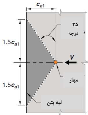
پلان ب- شکست مخروطی بتن در برش
