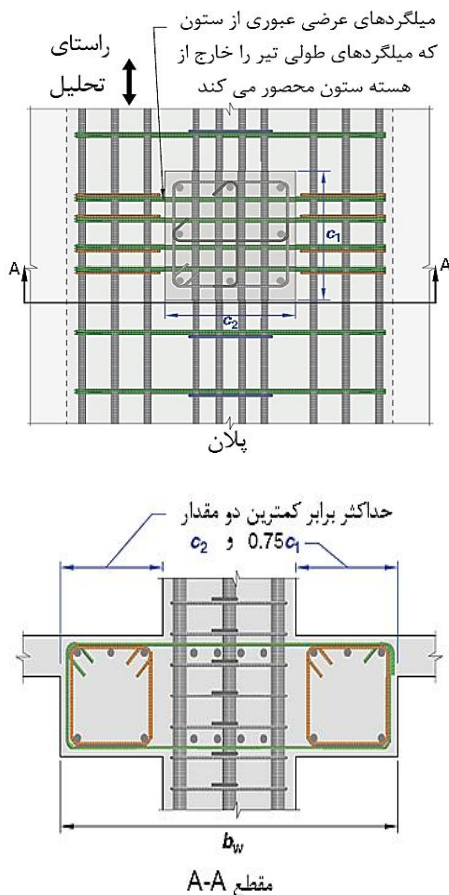
شکل ۲۰-۵ حداکثر عرض موثر در تیرهای پهن و آرماتور عرضی مورد نیاز
