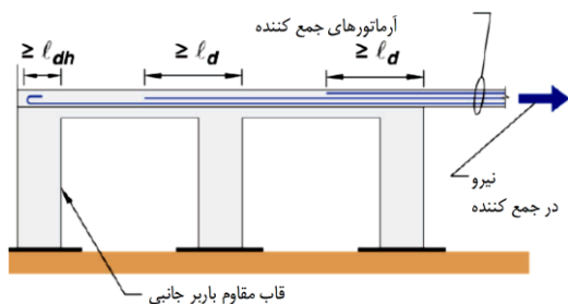
شکل ۱۴-۸ مسیر انتقال نیرو از جمع‌کننده به اجزاء قائم سیستم باربر جانبی
