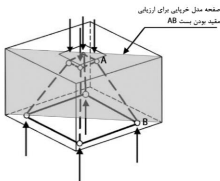
شکل ۱۰-۲۲ صفحه مدل خرابایی برای ارزیابی مقید بودن بست AB در مدل خرابایی سه بعدی یک سرشمع بتن آرمه
