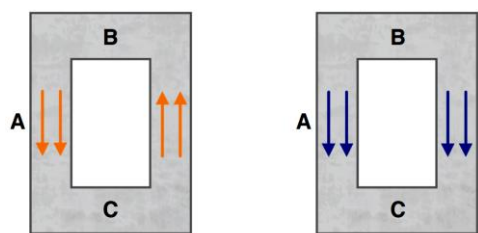
تنش‌های برشی ناشی از برش (جعبه‌ای) الف - مقطع توخالی
